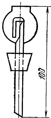
Затвор Геккеля
